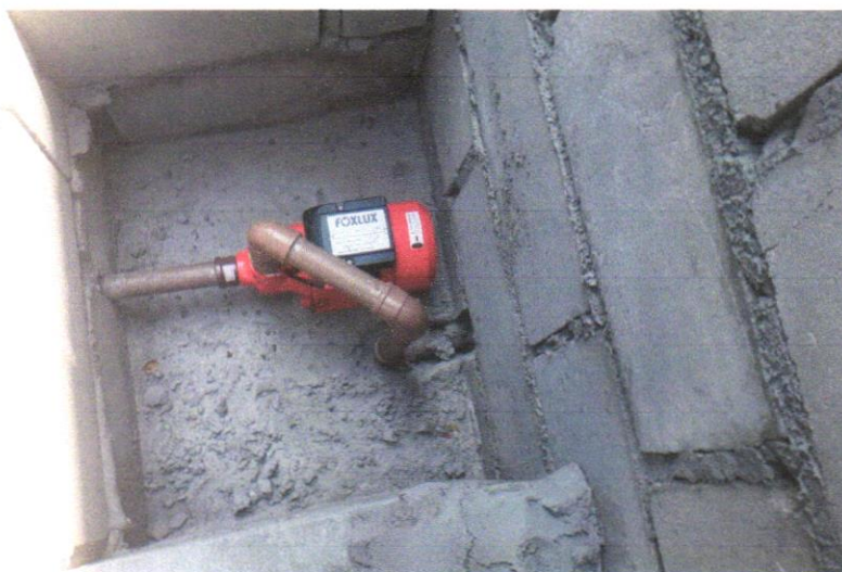
Foto 21 -BOMBA CENTRÍFUGA, MONOFÁSICA, 0,5 CV OU 0,49 HP, HM 6 A 20 M, Q 1,2 A 8,3 M3/H -
